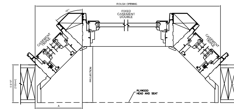
45° METAL CLAD CASERMENT 6 9/16" (166mm)
