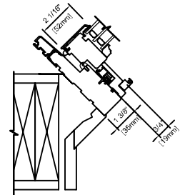
45° METAL CLAD CASERMENT 6 9/16" (166mm)
