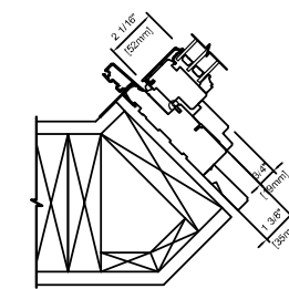
45° METAL CLAD CASEMENT 6 9/16\" (166mm)
